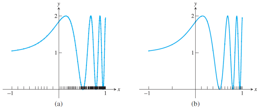
Figura 4: Cuadratura adaptivă aplicată funcției f(x) = 1 + \sin e^{3x} .
